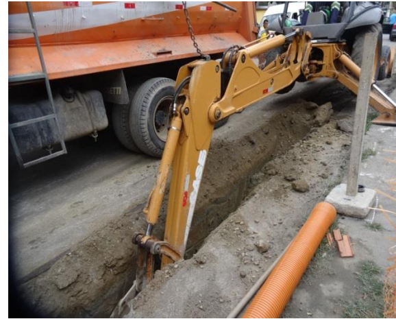
Execução de rede coletora Sub Bacia SR 2 (Sistema Sarapuí)
